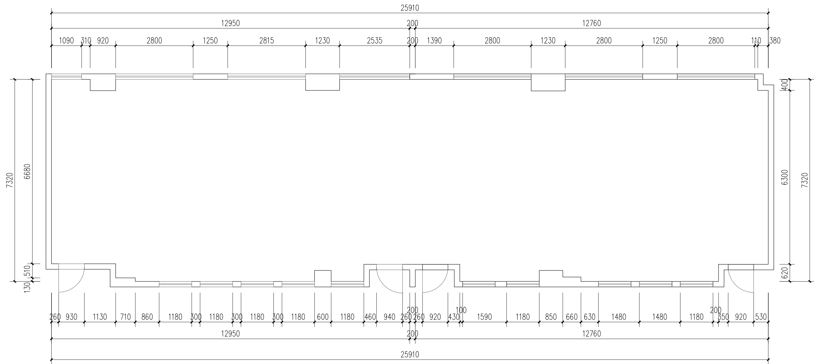
规划布置图
