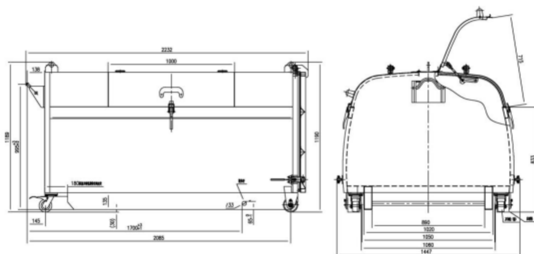
说明: 1. 图中尺寸除特殊标注外均为mm。
