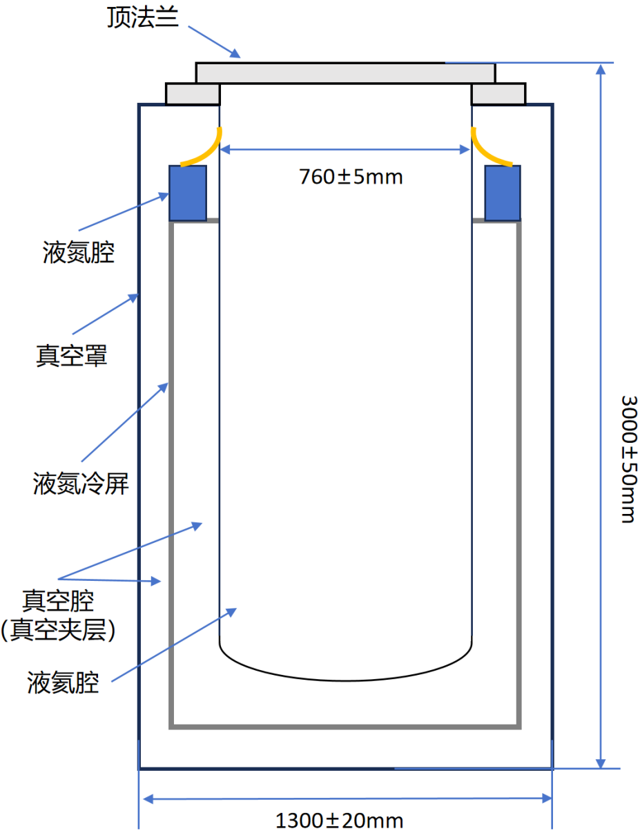
附图 1：（标段一）磁体敞口杜瓦系统的主体尺寸及结构示意图
