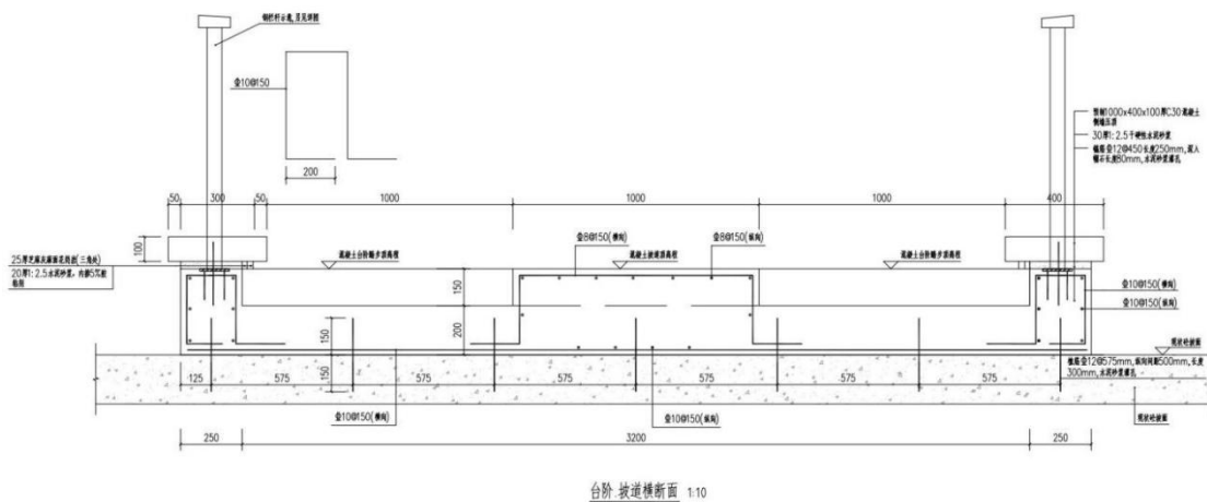
台阶坡道横断面图
