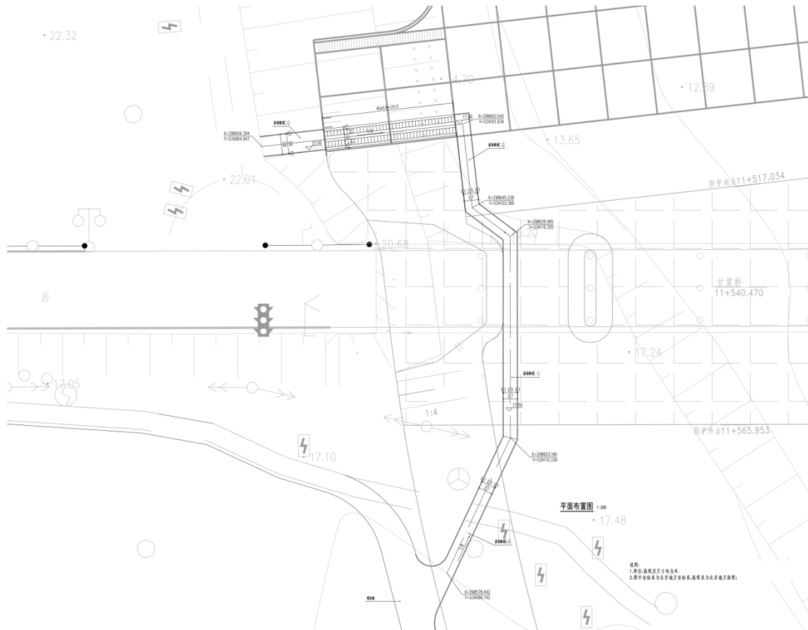
大运河森林公园至甘棠闸下步道连通平面布置图
