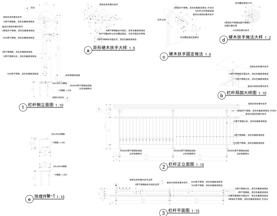
栏杆做法详图
