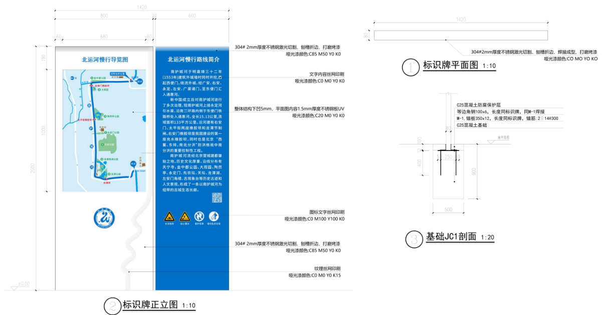
绕行导视牌样式示意图
