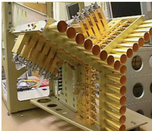
图2 一个卫星上搭载的天线阵列，形成综合孔径干涉
