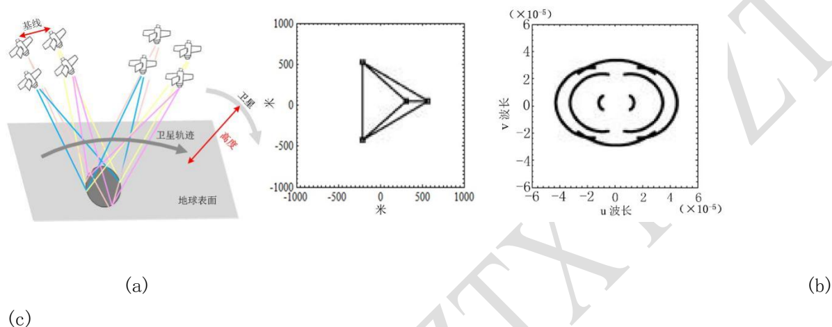
图1 小卫星编队综合孔径干涉稀疏成像示意图，(a)是小卫星编队对地成像图，(b)是小卫星编队几何构型，(c)是该编队构型在频域内（UV平面）的采样点分布。
