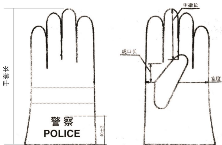
图2 成品手套主要部位测量示意图
