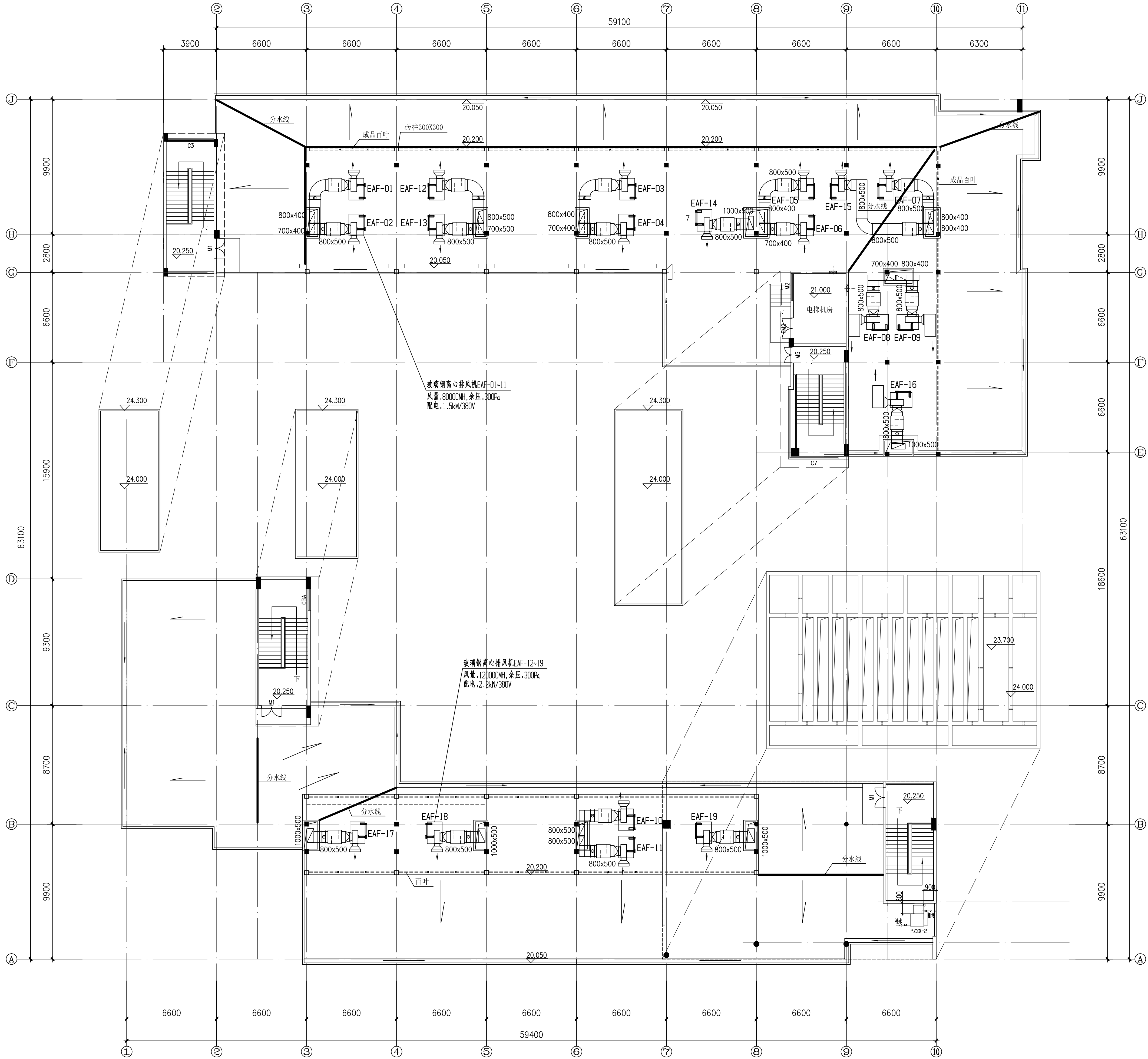
屋面风机布置图
